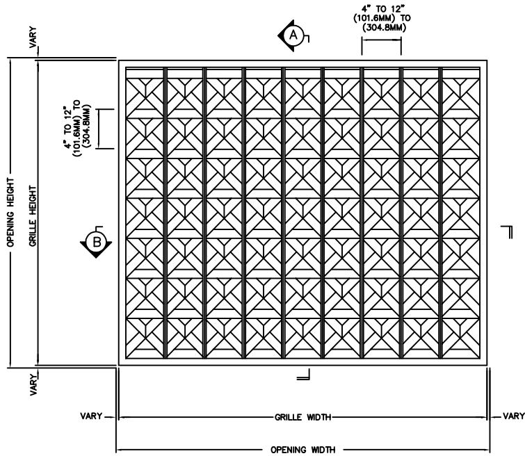
ELEVATION
