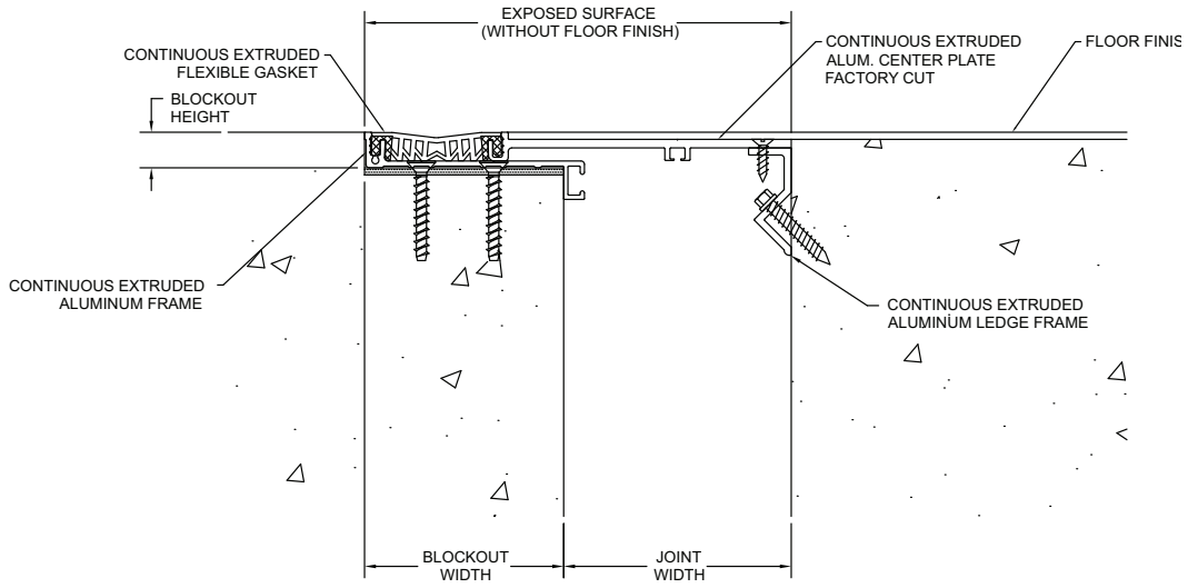
GTR-M (TYP.)
