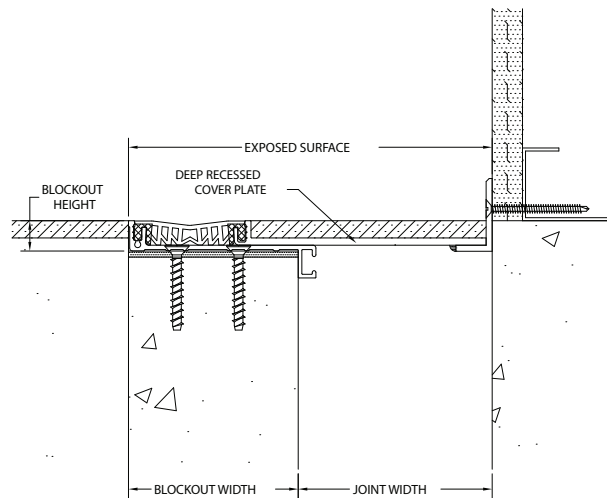
GTRW-D (TYP.)
