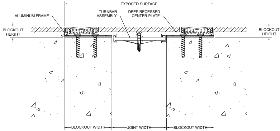
GTR-D (TYP.)
