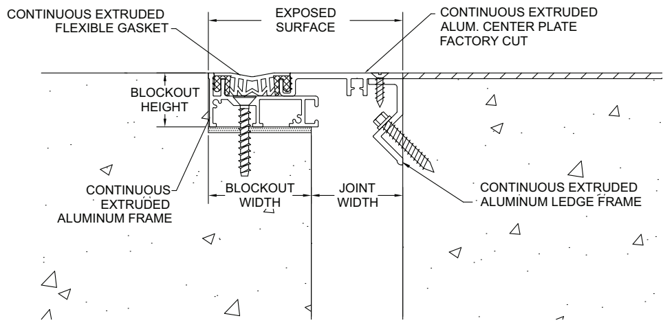
DGTP-M (TYP.)
