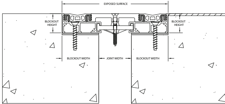
DGTP-HD (TYP.)
