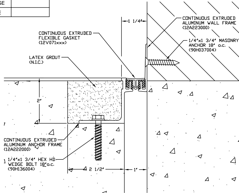
GFTW-100 X 2"
