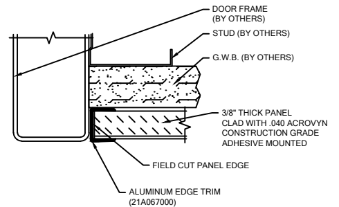
ALUMINUM EDGE TRIM QTY.: _____
