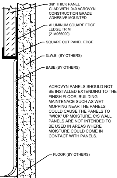
ALUMINUM SQUARE EDGE LEDGE TRIM QTY.: _____
